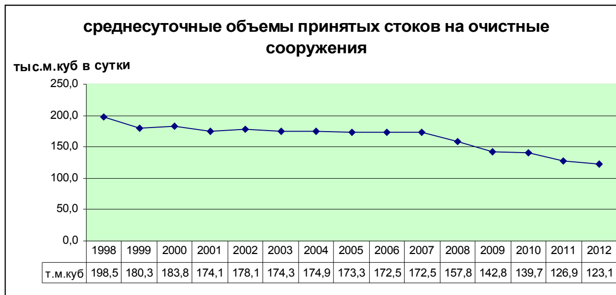
Рис. 18 – График среднесуточных объемов приняты стоков на очистные сооружения
