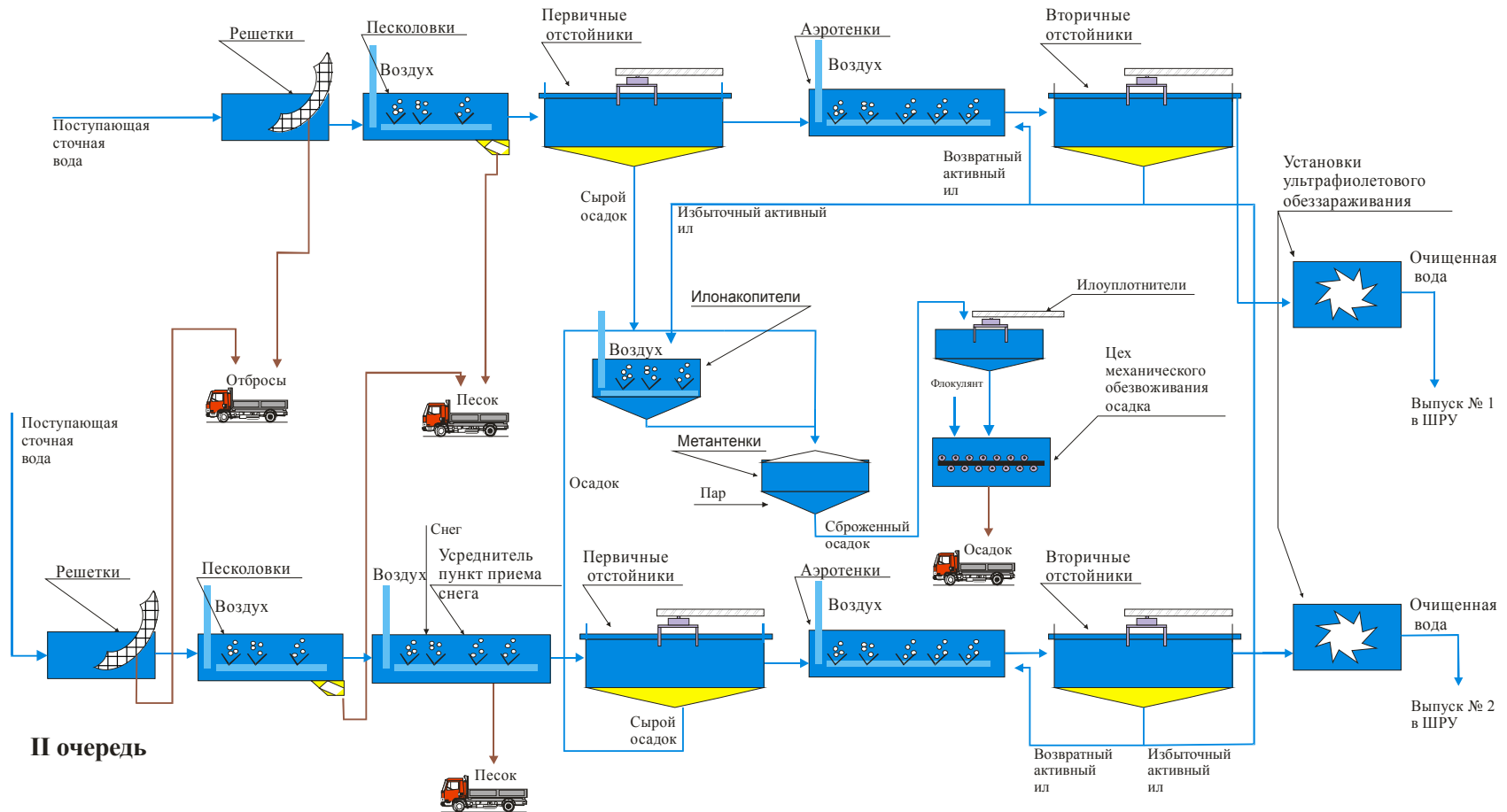
Рис. 16 – Технологическая схема КОСК ПБУ
