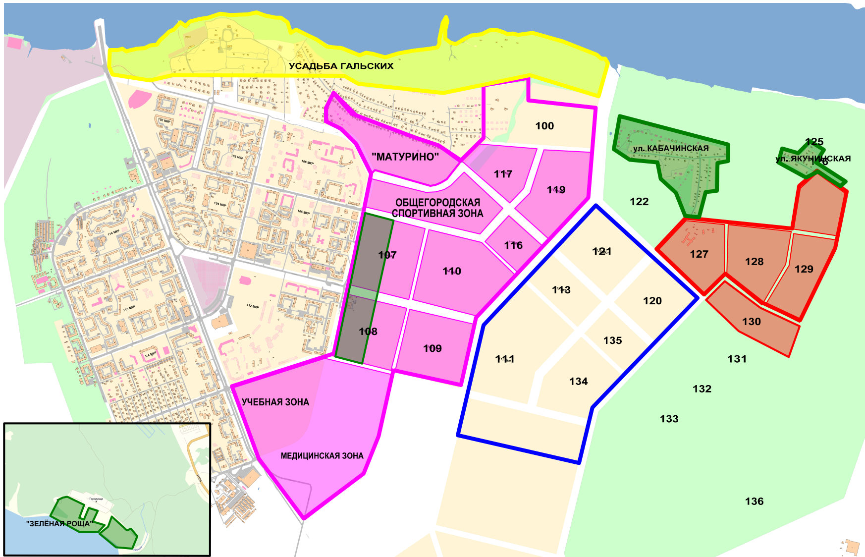
Рис. 12 - Схема планируемого размещения объектов централизованных систем водоснабжения и водоотведения Зашексинского района
