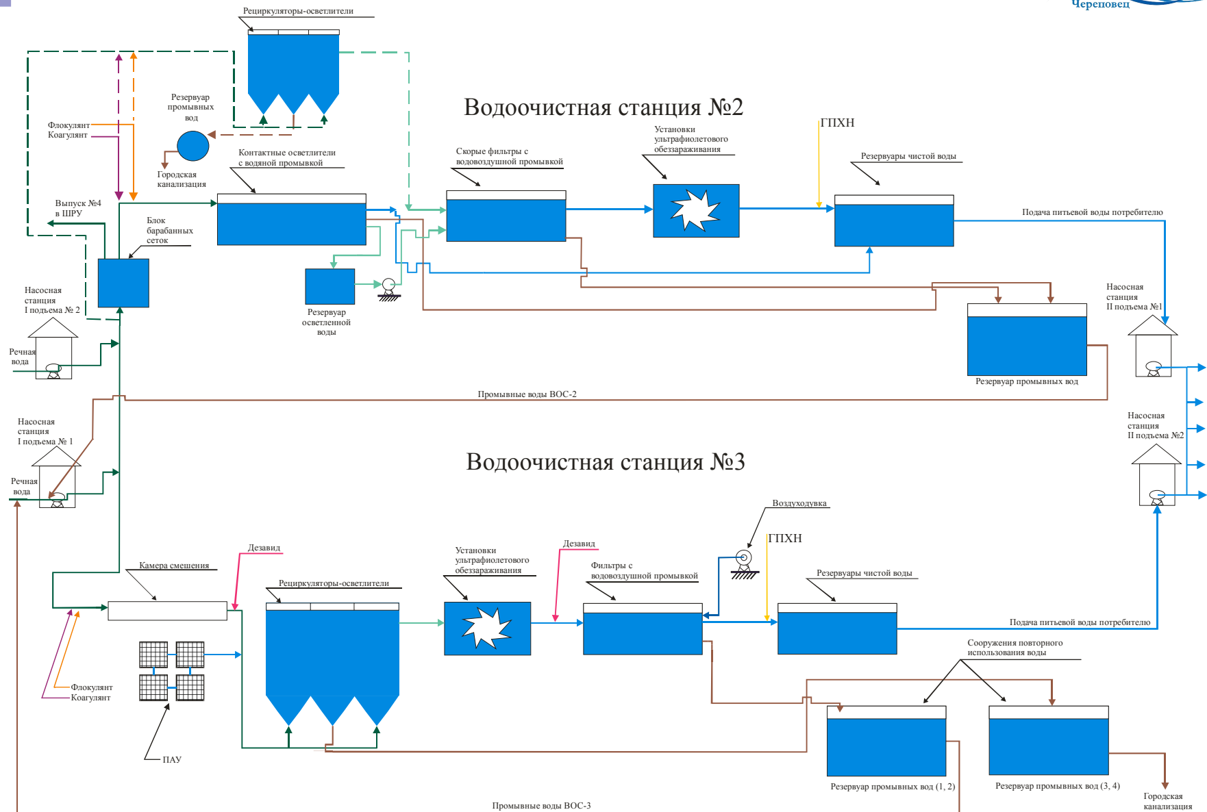
Рис. 2 Принципиальная схема водоподготовки на КВОС города Череповца
