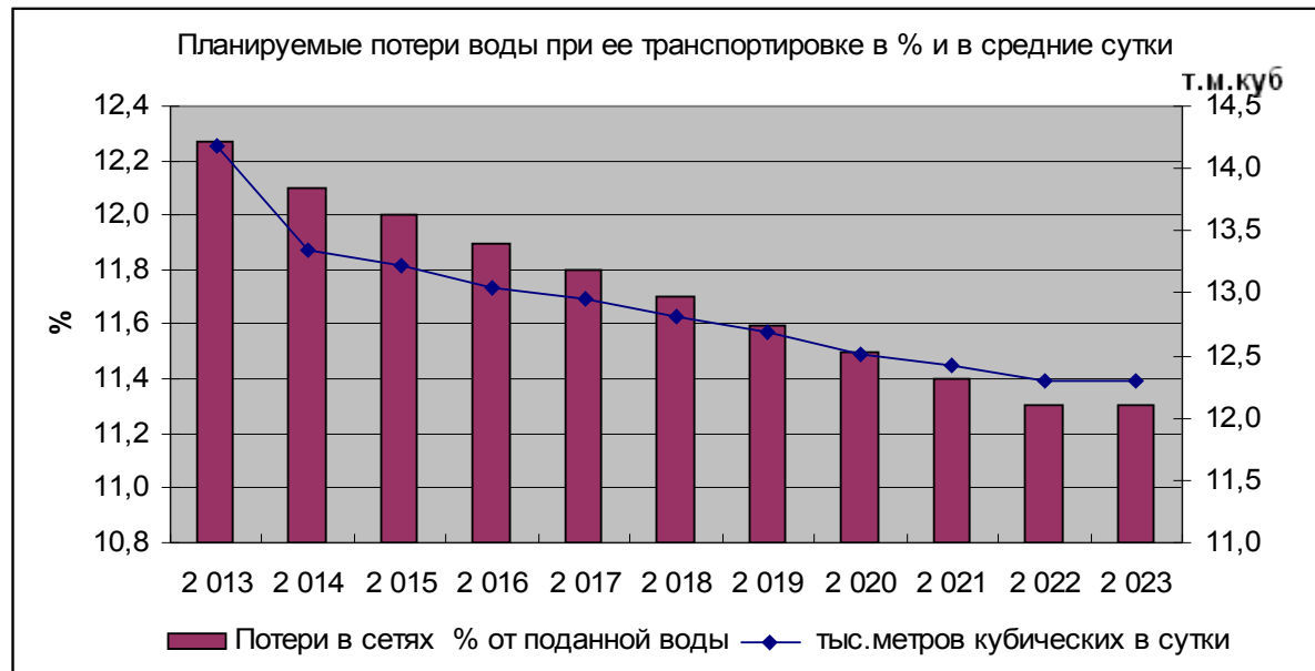
Рис.10 – График планируемых годовых потерь воды при ее транспортировке
