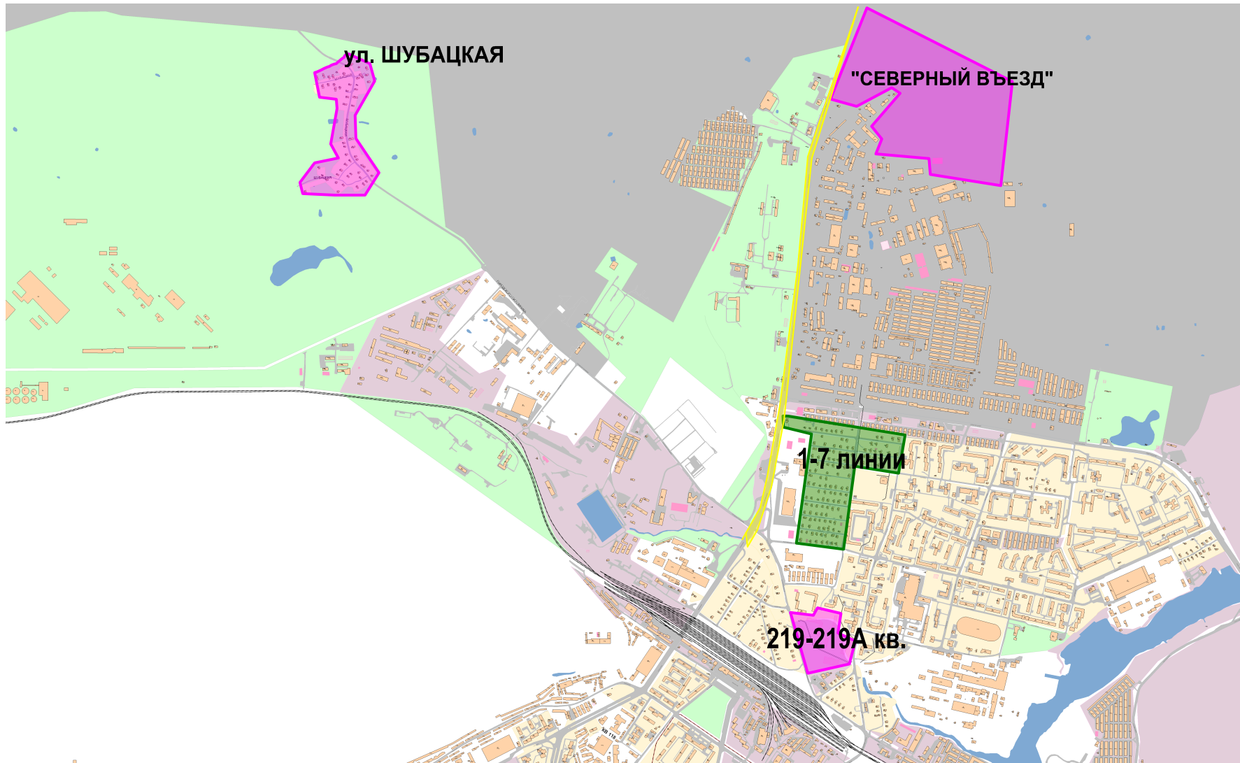
Рис. 15 - Схема планируемого размещения объектов централизованных систем водоснабжения и водоотведения Северного района
