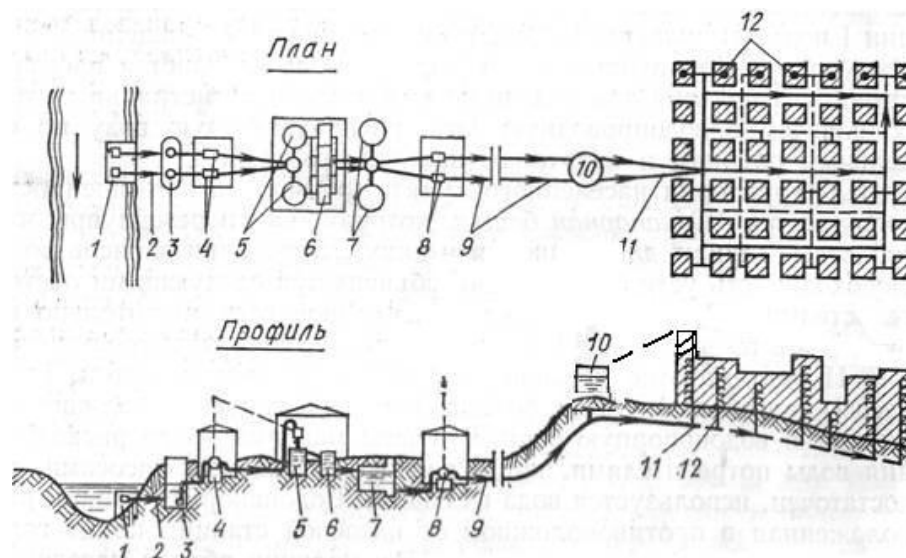
Рис.1. Структура системы водоснабжения г.Череповца
