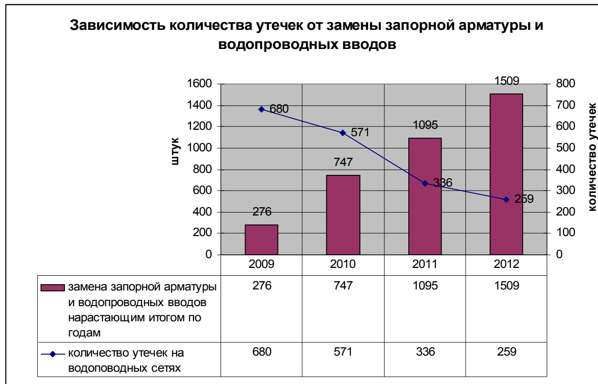
Рис. 3 - График зависимости количества утечек от замены запорной арматуры и водопроводных вводов
